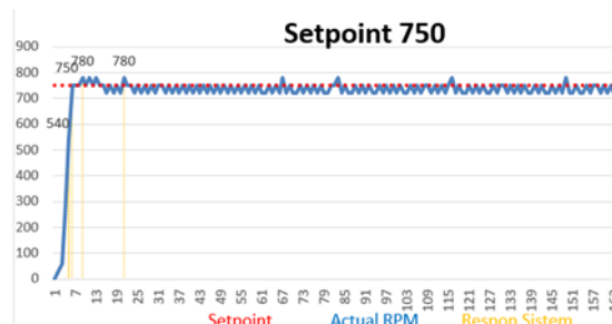
Gambar 10. Grafik Respon Setpoint 750.
