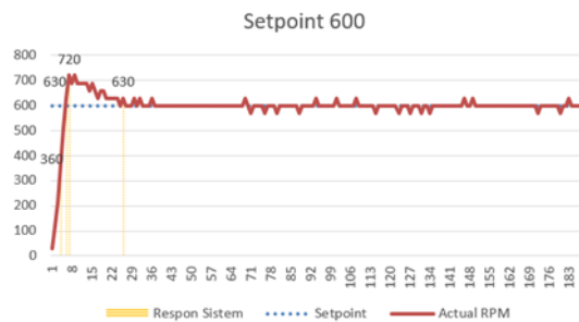
Gambar 9. Grafik Respon Setpoint 600.
