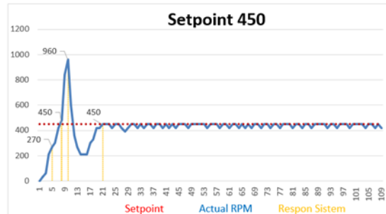
Gambar 8. Grafik Respon Setpoint 450.
