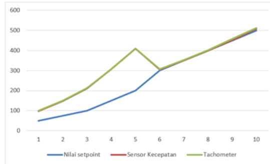
Gambar 4. Grafik Pengujian Sensor Kecepatan dengan Tachometer
